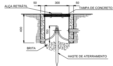
CORTE AA'
