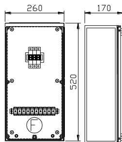
CAIXA PARA BARRA DE EQUIPOTENCIALIZAÇÃO PRINCIPAL (BEP) TIPO (POLIMÉRICO)
